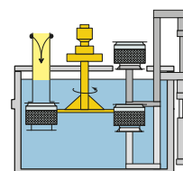
Карусельный закалочный бак
